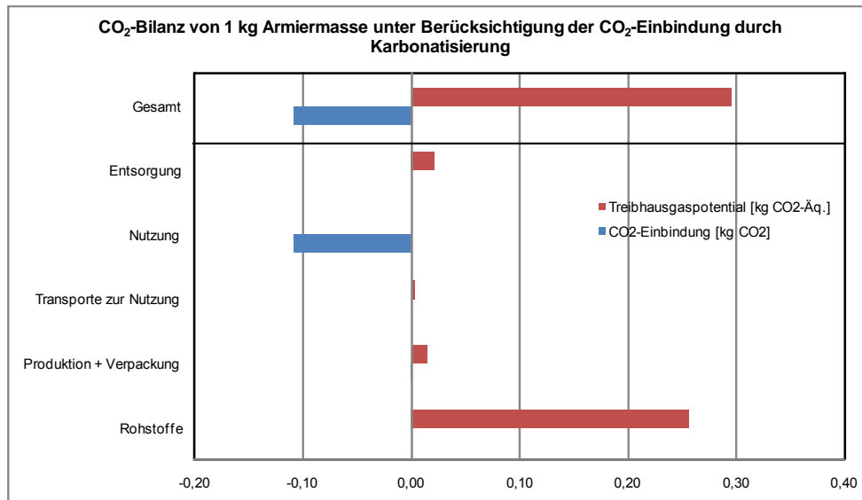
Abbildung 7-6: CO 2 -Bilanz von 1 kg Armiermasse CT-186M unter Berücksichtigung der CO 2 -Rückbindung durch Karbonatisierung
