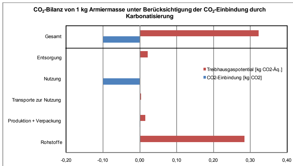
Abbildung 7-7: CO 2 -Bilanz von 1 kg Armiermasse CT-190 unter Berücksichtigung der CO 2 -Rückbindung durch Karbonatisierung
