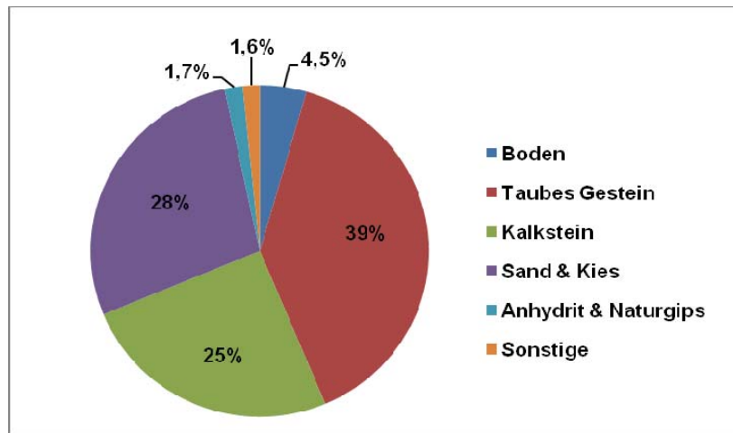
Abbildung 8-3: Aufteilung nicht erneuerbarer stofflichen Ressourcen bei der Herstellung von 1 m³ bewehrtem Hebel® Porenbeton inklusive Vorketten
